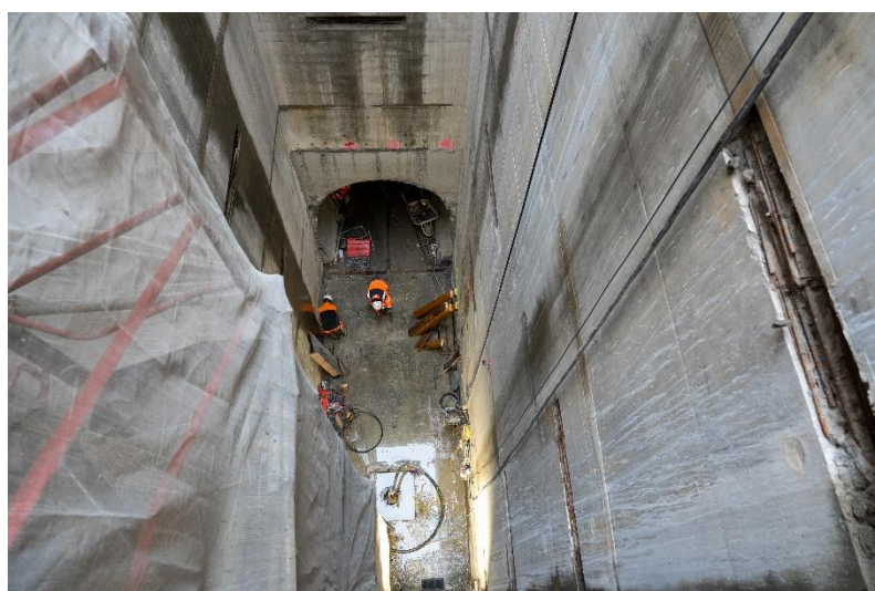
Puits Ferdinand Fauré – rameau de connexion ©MXR Communication – Tisséo Ingénierie Janvier 2026
