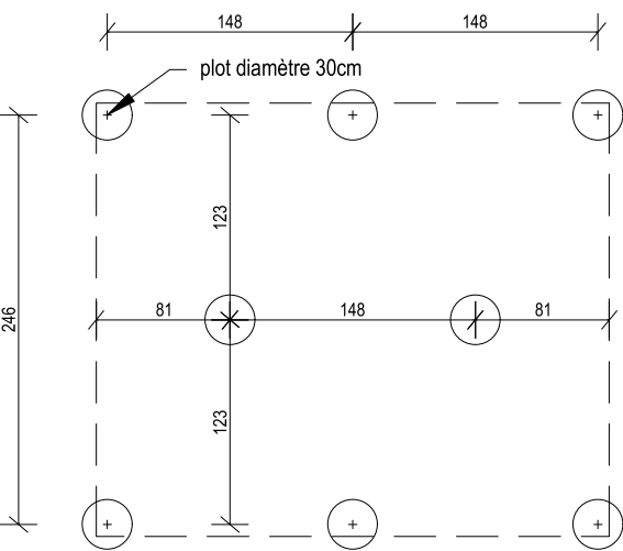
PLAN D'IMPLANTATION DES PLOTS BÉTON
