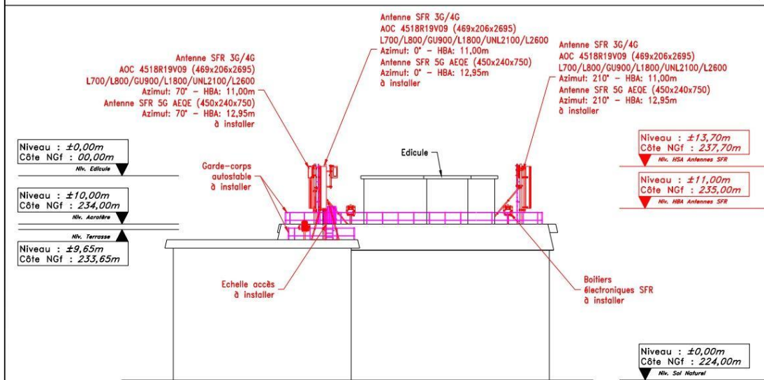
Vue A
