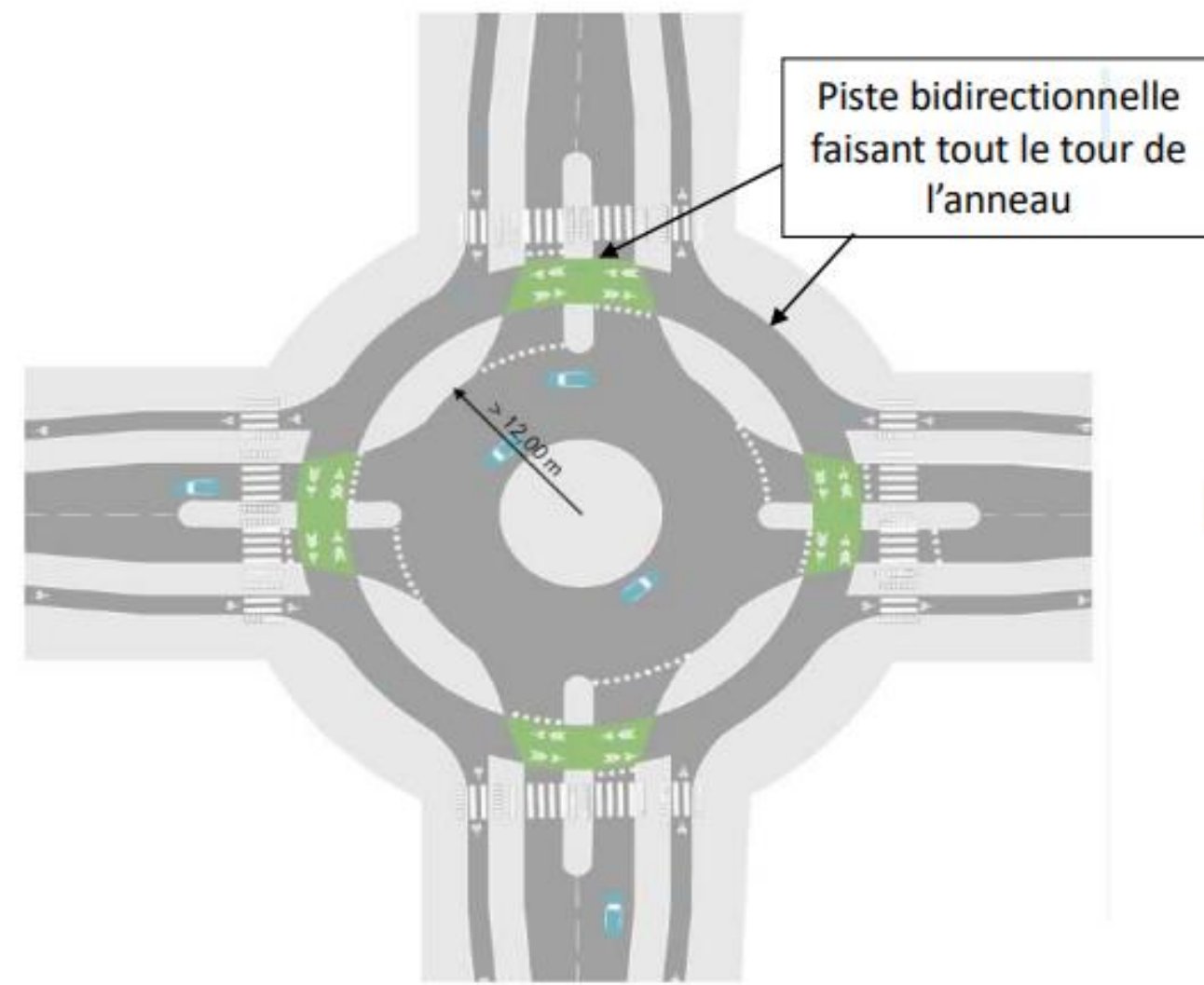
Traitement des grands giratoires type « Cerema »
