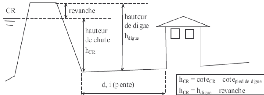
Extrait de l'étude CETE Med : paramètres pris en compte dans les simulations de rupture de digues
